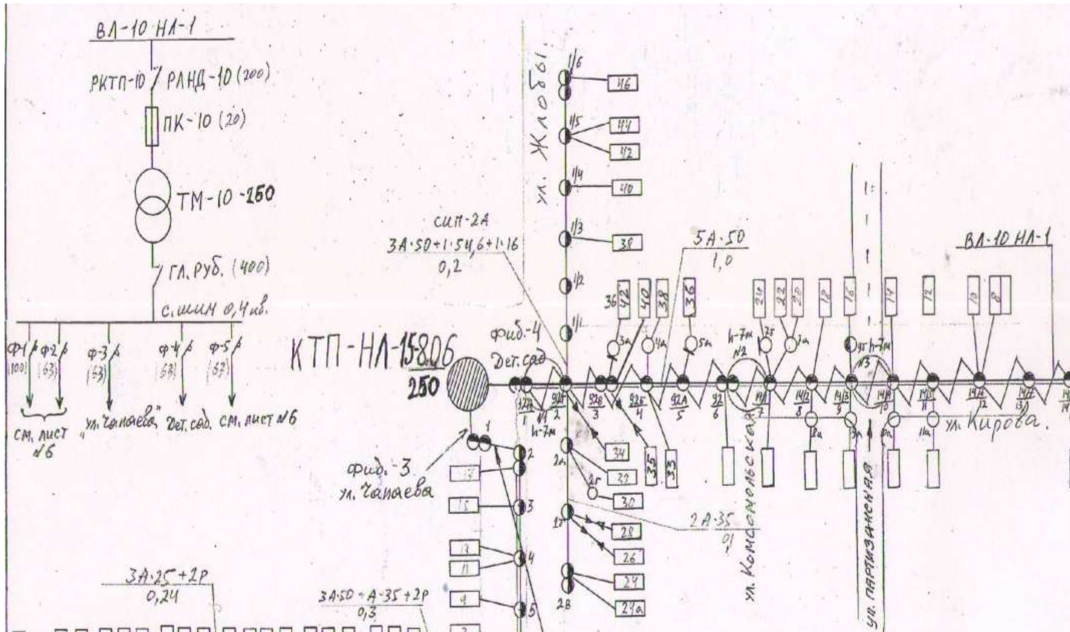
Обосновывающие материалы. Схема электроснабжения (лист № 7) ст. Новолешковская. Масштаб 1:5000
