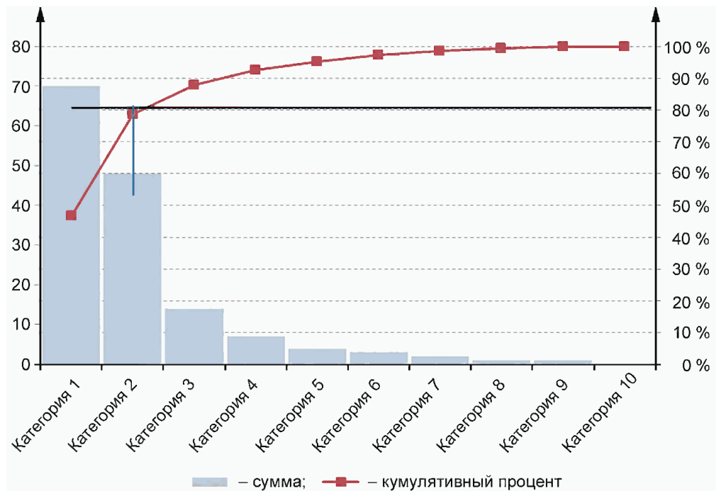
Рисунок Б.16 - Пример диаграммы Парето
