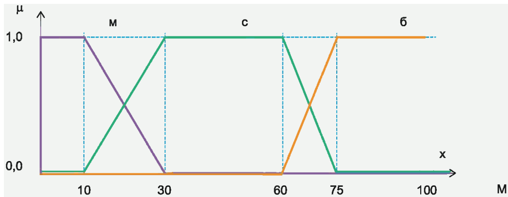
Рисунок Б.13 - Пример нечеткого понятия "несколько" с тремя термами (значениями) лингвистической переменной "ущерб"
